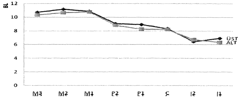
Grafik 1: Üst ve Alt Dişlerin BL Ortalamaları (mm)
