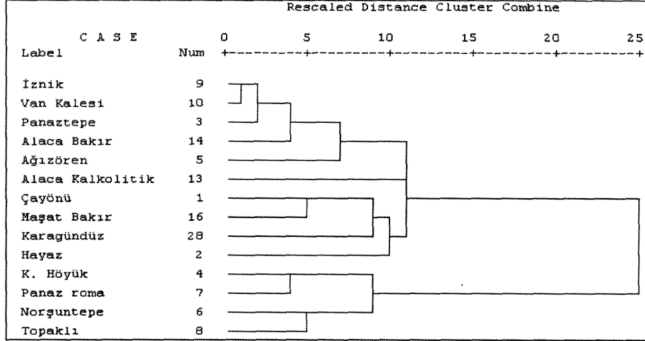
Grafik 3: Eski Anadolu Toplumlarının Cluster Analizi
